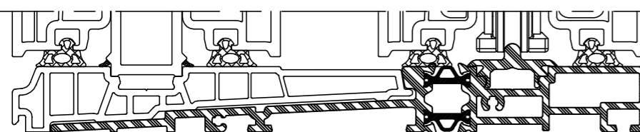
Soglia "Bassa" 20 mm - DI SERIE -
