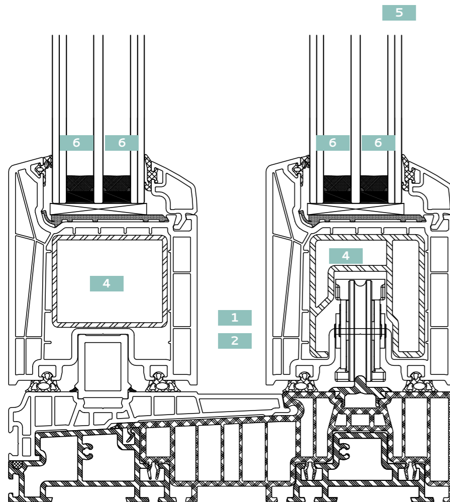
Soglia "Alta" 48 mm da incasso
