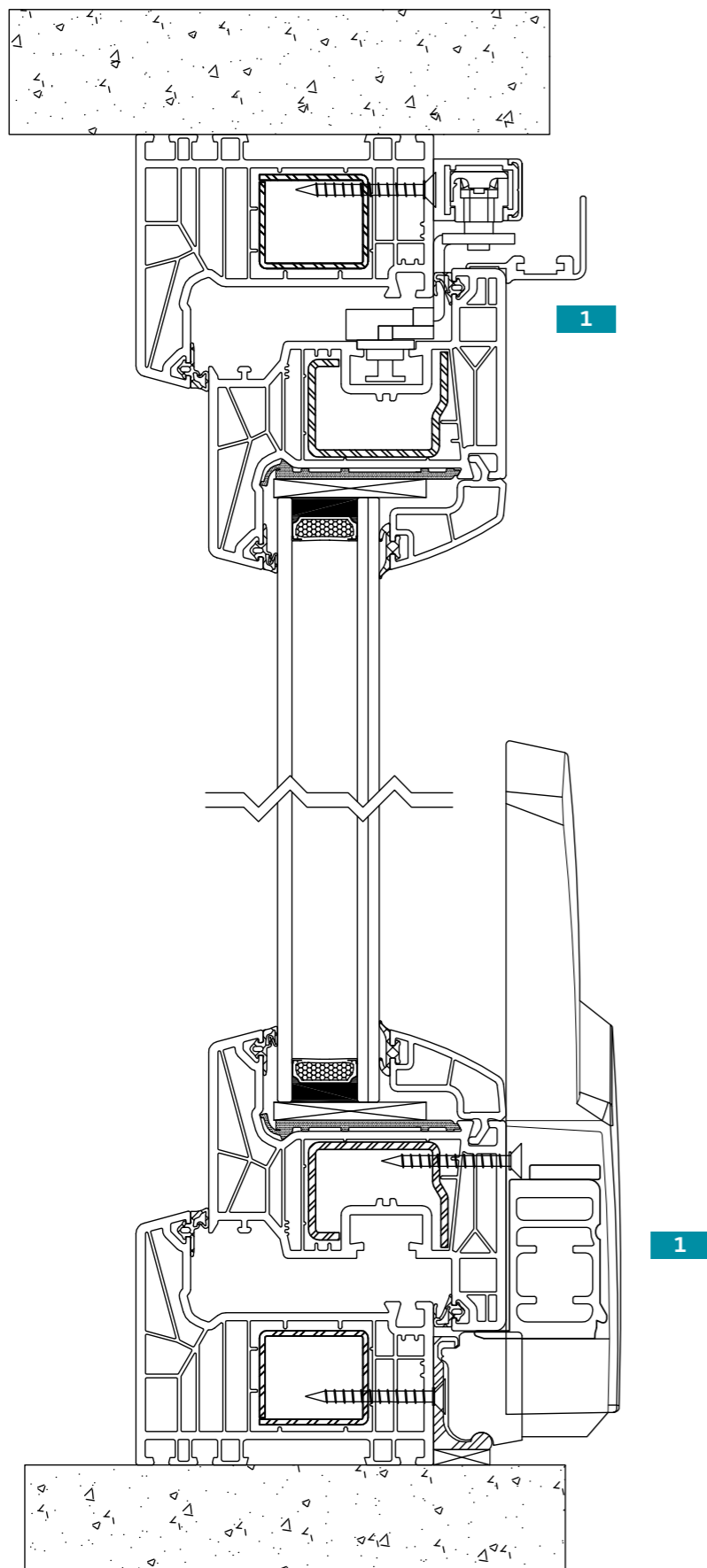
1 Guida e meccanismo
