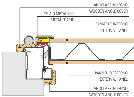
NODO TELAILO METALLICO METAL FRAME NODE
