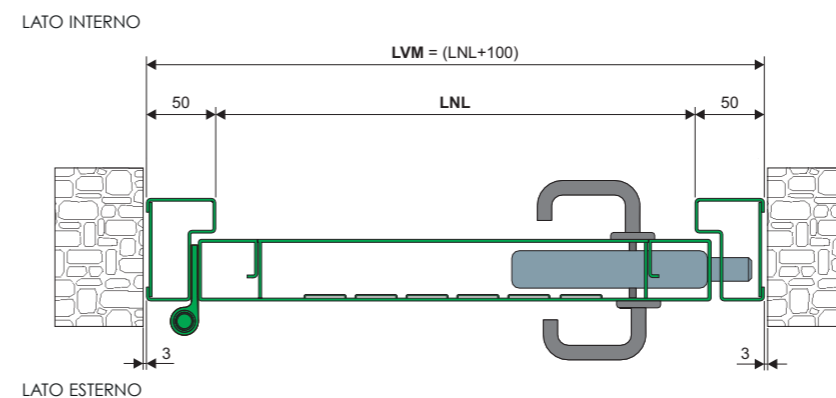
SEZIONE TRASVERSALE
