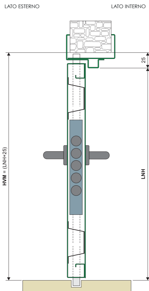
SEZIONE LONGITUDINALE
