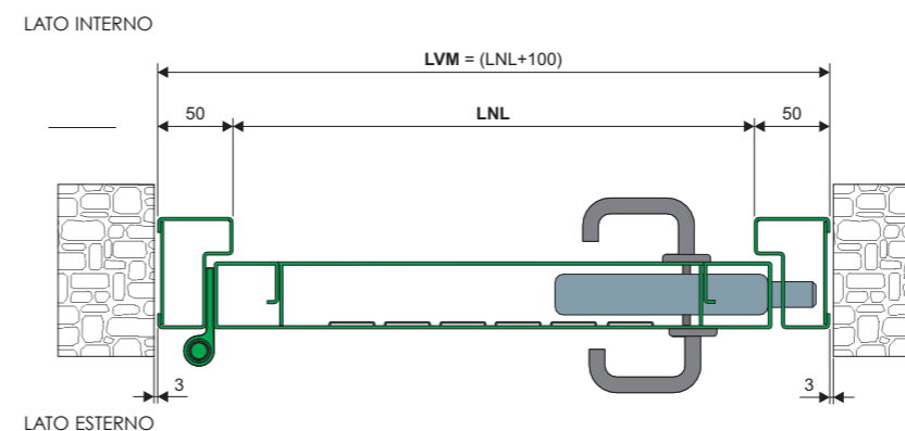
SEZIONE TRASVERSALE
