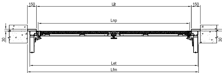
SEZIONE ORIZZONTALE HORIZONTAL SECTION
