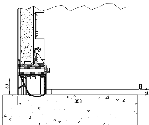
Dettaglio soglia per porta senza portina pedonale Thershold detail for door without pedestrina door
