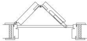
LIBRO 1/2 + 1/2 SISTEMA 2 SX
