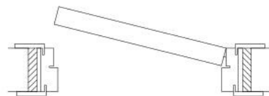
CERNIERE A SCOMPARSA DX
